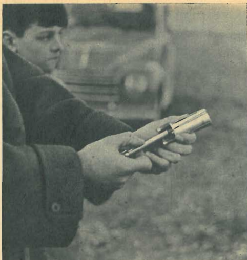
A rifornimento avvenuto, si chiude il Jetex mettendo in tensione le molle.
